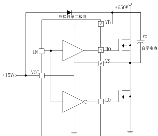
图 8-3. EG2184S 自举电路结构
