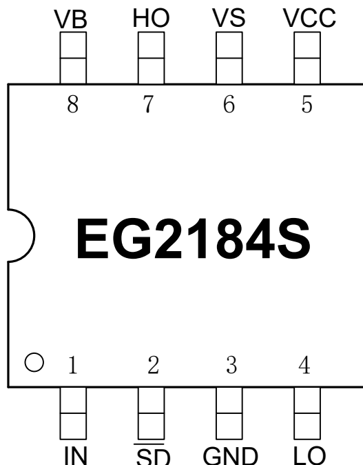
图 4-1. EG2184S 管脚定义
