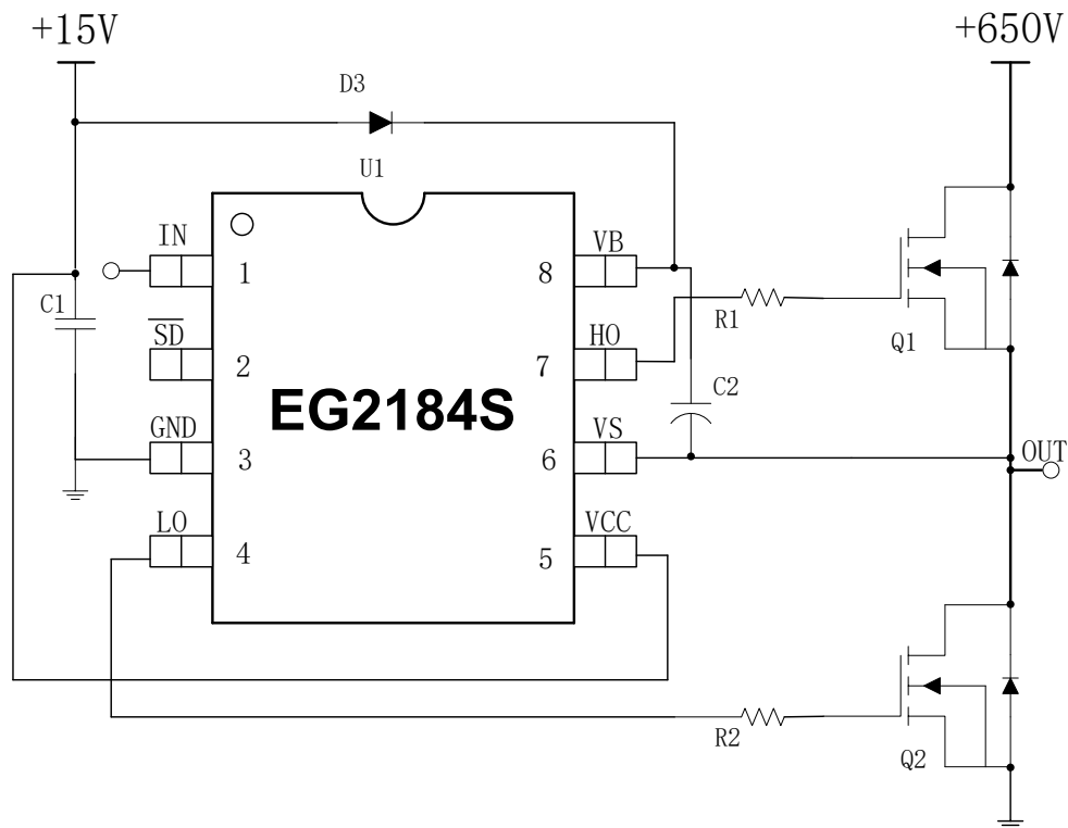
图 6-1. EG2184S 典型应用电路图
