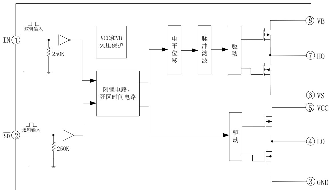
图 5-1. EG2184S 内部电路图
